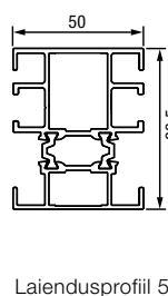
Laiendusprofiil 50 mm
