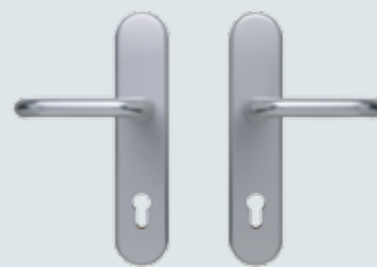
Lingikomplekt, ES 1, pikk katteplaat, eurosüdamiku valmidus, roostevaba teras
