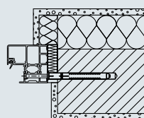
Karpleng Paigaldus müüritisse Tüübepaigaldus
