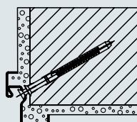
Spetsiaalne nurkleng Tüübepaigaldus läbi lengi
