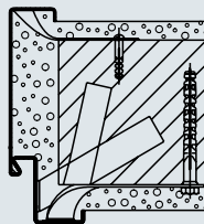
Põski ümbritsev leng Paigaldus müüritisse Müüriankrud
