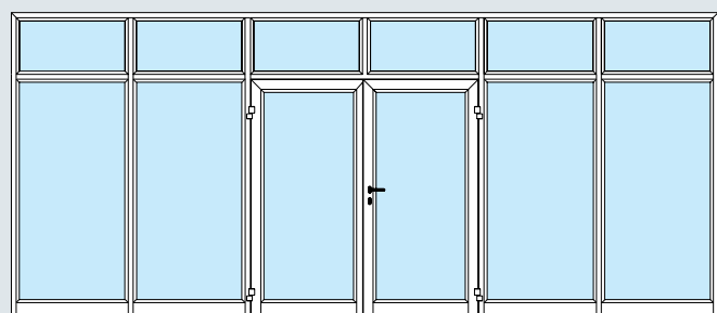
Motiiv 102 koos küljeosade ja framuugidega
