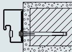
Karpleng Paigaldus müüritisse Tüübelmontaaž
